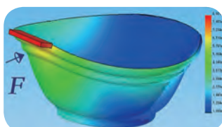
フチ部への衝撃をシミュレーション解析
