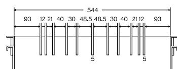
⑭ PPコンテナ PC-37B用仕切り板 〈AKV-Q2〉 8-0156-1401 大 555×180×厚さ5 ¥1,100 8-0156-1402 小 355×180×厚さ5 ¥820 材質: ポリプロピレン
