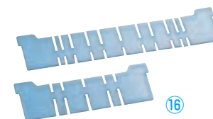
⑯ PPコンテナ PC-27B用仕切り板 〈AKV-Q0〉 8-0156-1601 大 555×130×厚さ5 ¥900 8-0156-1602 小 355×130×厚さ5 ¥700 材質: ポリプロピレン
