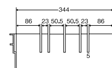
⑯ PPコンテナ PC-27B用仕切り板 〈AKV-Q0〉 8-0156-1601 大 555×130×厚さ5 ¥900 8-0156-1602 小 355×130×厚さ5 ¥700 材質: ポリプロピレン
