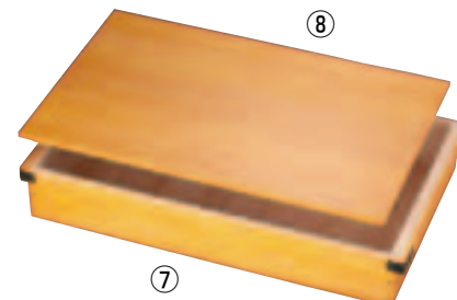
⑦ 木製 麺箱 (外面クリア仕上) 〈AMN-L1〉 8-0156-0701 ¥12,000 外寸: 580×345×H90 内寸: 530×320×H85
