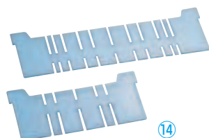
⑭ PPコンテナ PC-37B用仕切り板 〈AKV-Q2〉 8-0156-1401 大 555×180×厚さ5 ¥1,100 8-0156-1402 小 355×180×厚さ5 ¥820 材質: ポリプロピレン
