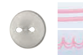
⑨ 口金 二穴 #43 注文コード 直径×高さ 絞り口(最大) 標準価格 CD 05-0387-0901 φ18×H29mm 約9mm ¥240 480048 材質/18-8ステンレス
