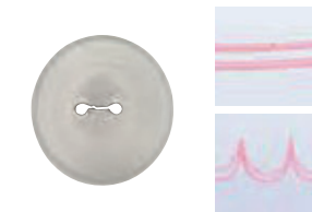
⑦ 口金 二穴 #41 注文コード 直径×高さ 絞り口(最大) 標準価格 CD 05-0387-0701 φ18×H33mm 約6mm ¥240 480046 材質/18-8ステンレス
