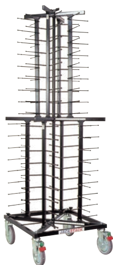
③ジャックスタック JS-072 7カ ページコード 商品コード 価格 1-2202-0301 5208200 ¥268,000
