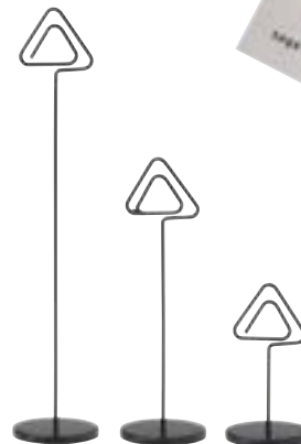
カードスタンド(トライアングル) SP-331 (大) ¥620 S:150×φ30(3)mm SP-332 (中) ¥580 S:100×φ30(3)mm SP-333 (小) ¥540 S:55×φ30(3)mm C:ブラック、Lot:10、※スチール
