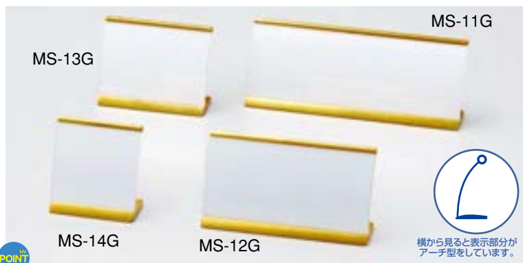
アルミカード立て&メニュー(アーチ型) C:ゴールド、Lot:10 MS-11G(大) ¥2,400 S:210×H88×40mm MS-12G(中) ¥2,000 S:150×H88×40mm MS-13G(小) ¥1,700 S:105×H88×40mm MS-14G(ミニ) ¥1,500 S:78×H88×40mm
